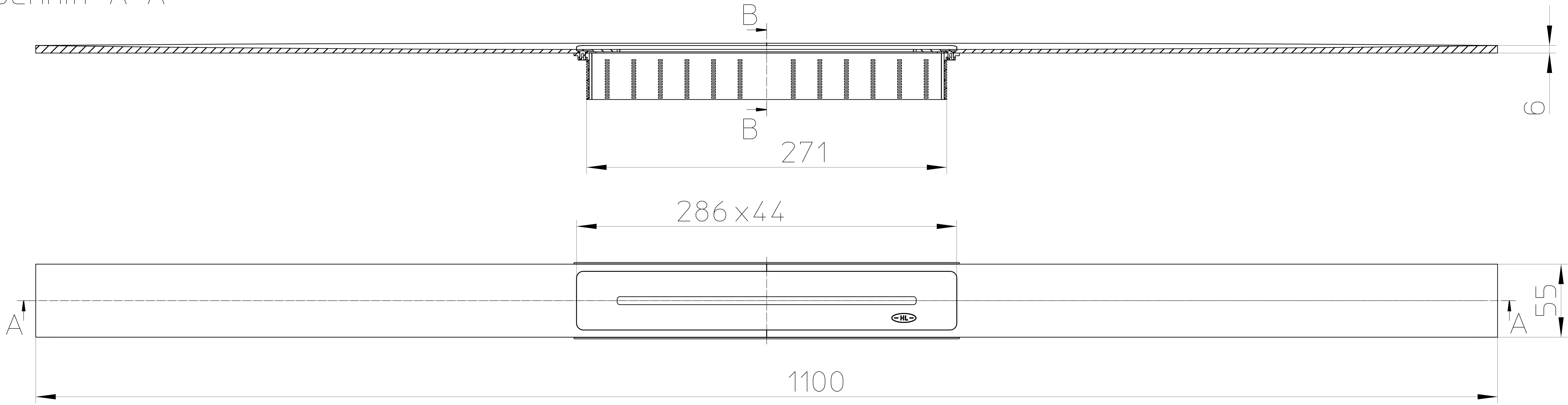
Schnitt A-A
