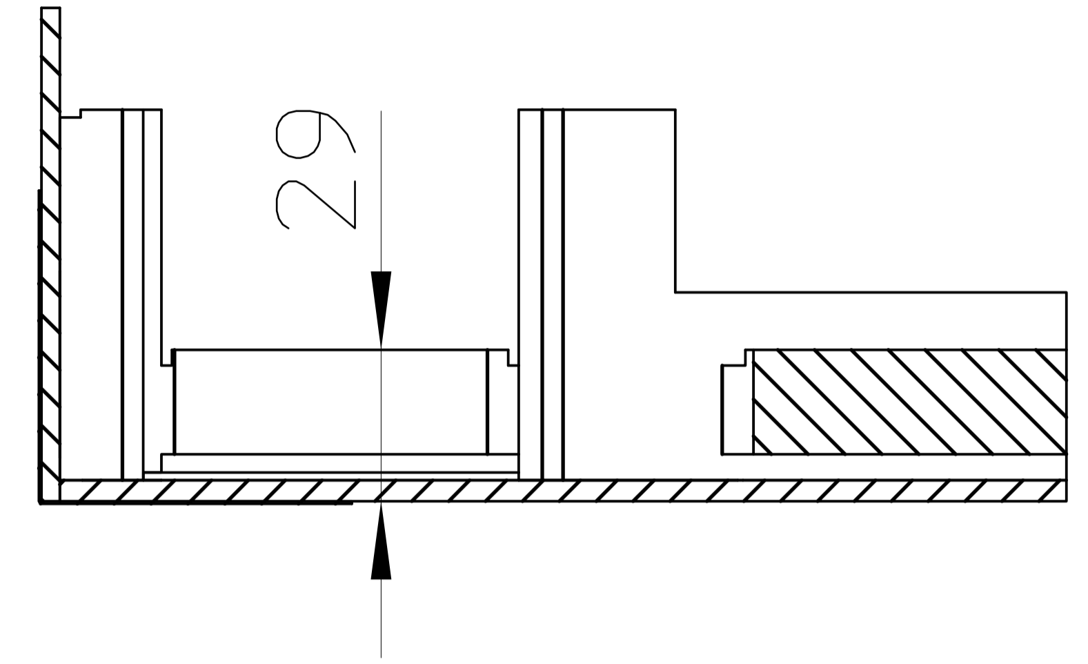
Schnitt A-A
